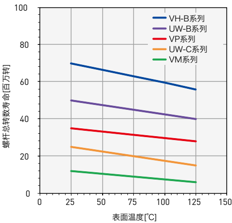
图14. 温度-螺杆总转数寿命特性
