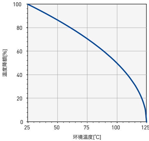
图5. 温度降额
