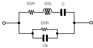
图7. 真空电容器的等效电路
