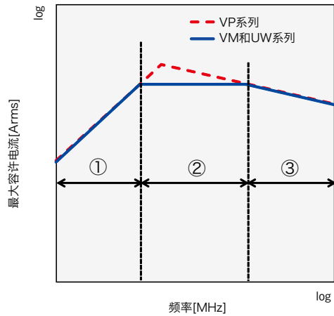
图4. 频率-最大容许电流特性
