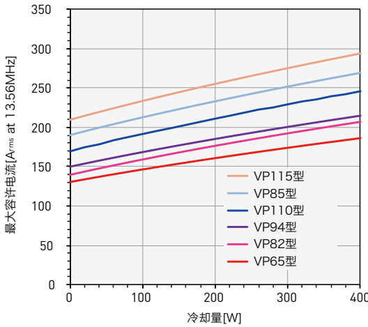
图6. 冷却量-最大容许电流特性
