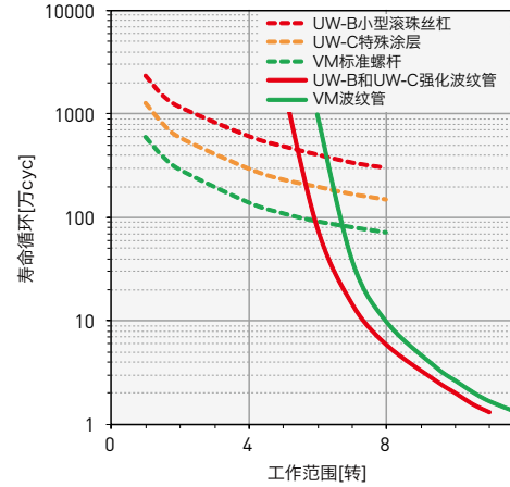
图16. 工作范围-寿命循环特性
