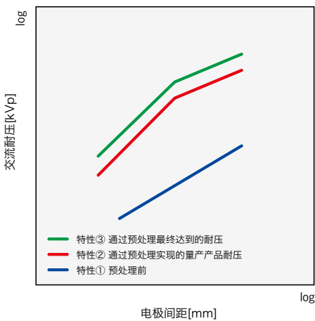
图2. 电极间距-耐压特性
