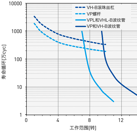
图15. 工作范围-寿命循环特性
