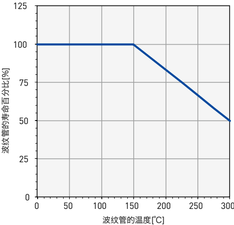
图12. 温度-波纹管寿命特性
