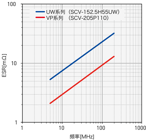
图9. ESR的频率特性示例
