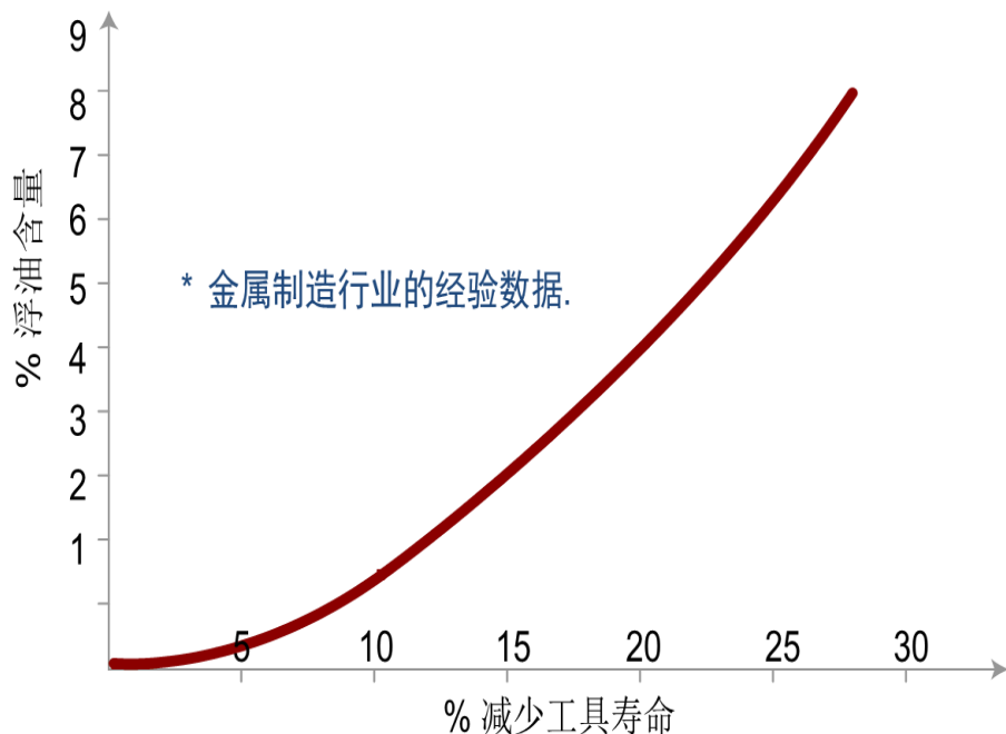
浮油与刀具寿命的关系
