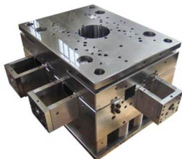
出口压铸模架
