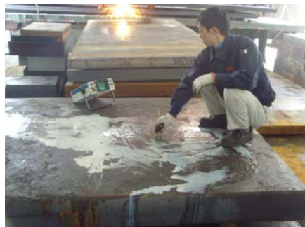
超声波探伤材料
