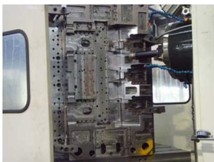
复杂注塑模架斜面加工
