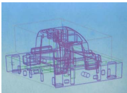
生成刀具路径
