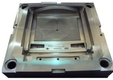
TV模架A板精成型
