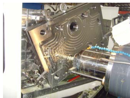
出口DME模架加工
