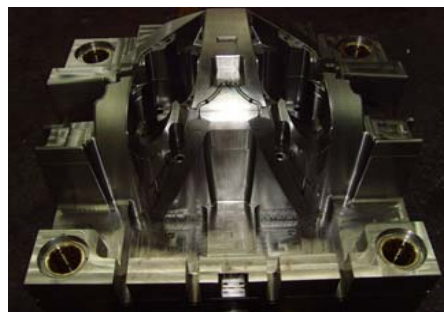
精成型车灯模架
